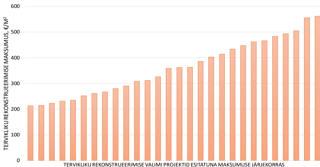
Joonis 30. Üksikelamute tervikliku rekonstrueerimise maksumus netopinna ruutmeetri kohta.
