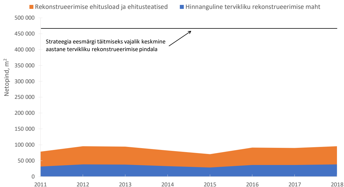
Joonis 21. Üksikelamute rekonstrueerimise ehitusload ja ehitusteatised netopindala alusel.
