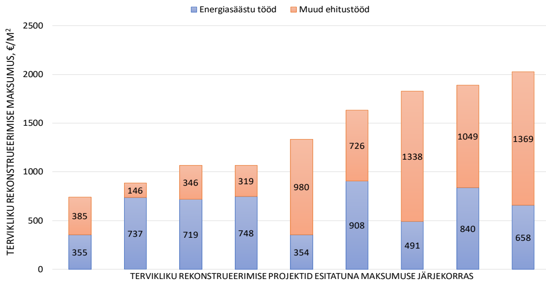
Joonis 32. Avaliku sektori hoonete tervikliku rekonstrueerimise maksumus netopinna ruutmeetri kohta.
