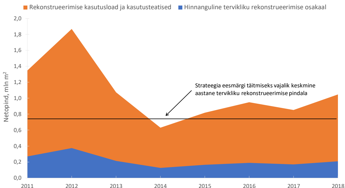
Joonis 29. Sisekliima tagamisega mitteeluhoonete rekonstrueerimise kasutuslood ja kasutusteatised netopindala alusel.
