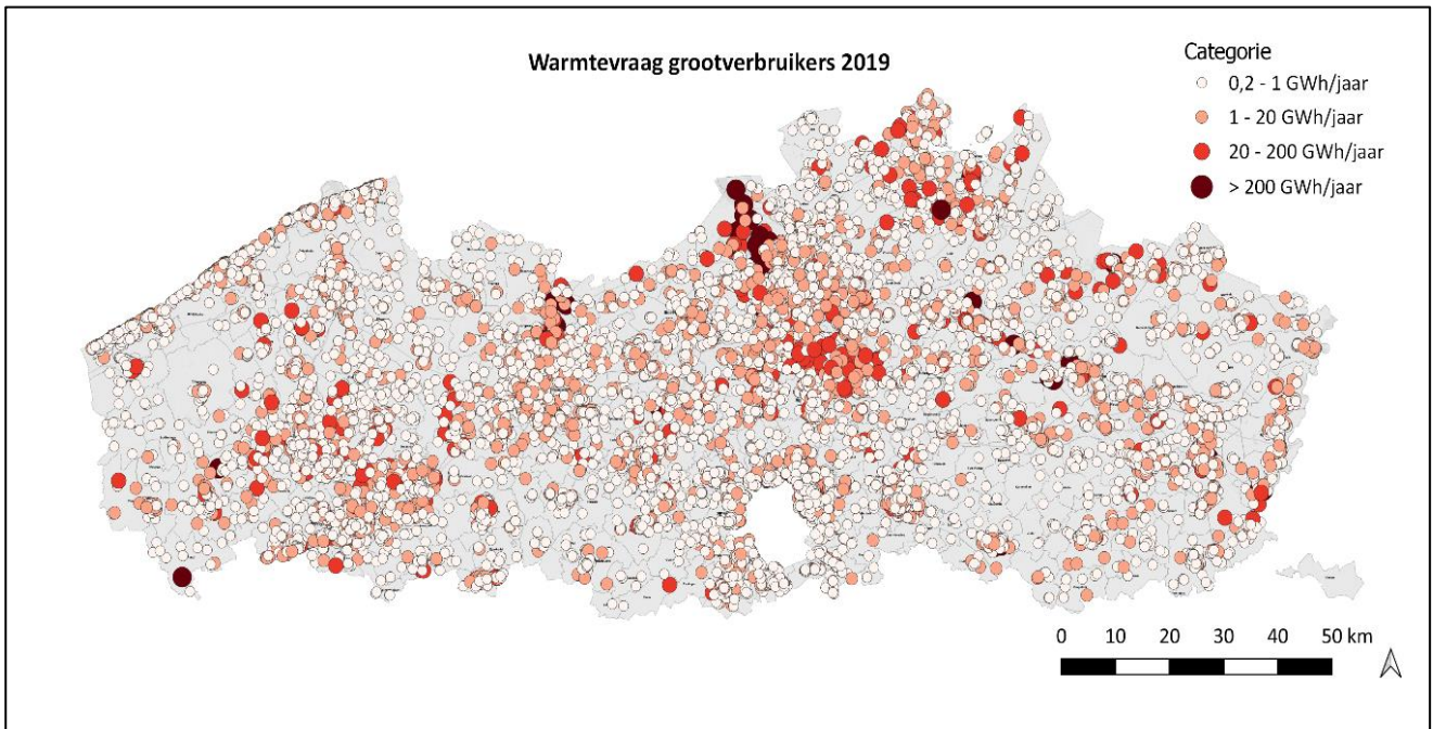
Figuur 10: Warmtevraag grootverbruikers 2019 (bron: Fluvius, IMJV)
