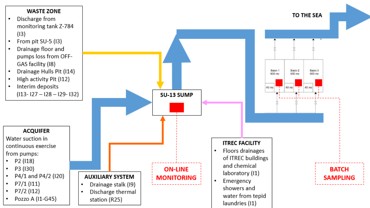
Figure 2. ITREC site drainages
