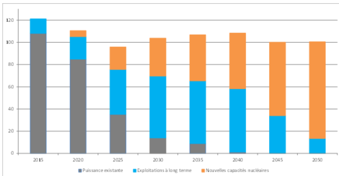
Figure 1 - Puissance nucléaire totale installée dans l'UE (GWe)
